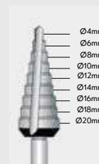
MÈCHE ÉTAGÉE N°1 - Ø4 - 20MM Réf. 6120 MÈCHE ÉTAGÉE N°2 - Ø4 - 30MM Réf. 6130
