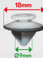
VB51505 AGRAFE MOULURE PB Megane II, Scenic III
