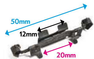
VB4000110 AGRAFE MÉTAL ENJOLIVEUR Trafic - Clio 3
