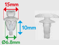
VB4000716 AGRAFE TOLE AUVENT
