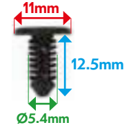
VB4000715 AGRAFE TOLE AUVENT
