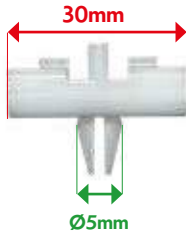
VB12036 AGRAFE VITRAGE R50, R52 et R53
