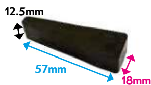
VB4000501 CALE CAOUTCHOUC Coccinelle (11-), Scirocco III (08-)
