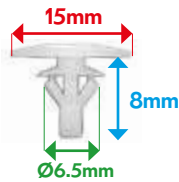
VB4000713 AGRAFE TOLE AUVENT
