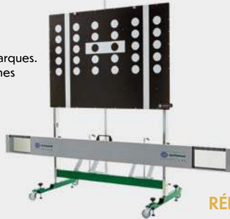
JEU DE TÊTES D'ALIGNEMENT RÉF. 8PZ015269-131
