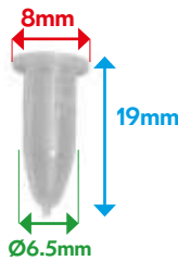
VB89427 TÉTINE DE PANNEAU DE PORTE Ulysse et Scudo
