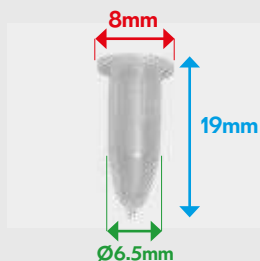
VB89427 TETINE DE PANNEAU DE PORTE 106, 205, 306, 309, 405
