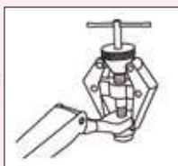
OUTIL DE DÉMONTAGE ESSUIE-GLACE frontaux montés avec vis et écrou. Après avoir dévissé la vis de fixation, positionner l'outil sur le bras d'essuie-glace et tendre uniformément jusqu'à ce que ce dernier se détache.
