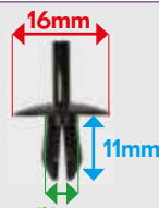
VB4000723 AGRAFE TOLE AUVENT
