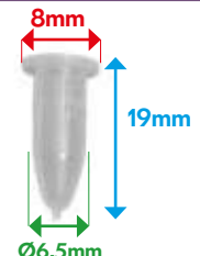
VB89427 TETINE DE PANNEAU DE PORTE AX, BX, Xantia, XM
