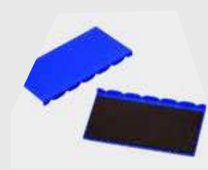
SET DE PROTECTION CARROSSERIE (2PCS) en plastique aimanté, protège contre le ponçage, l'accrochage et la peinture
